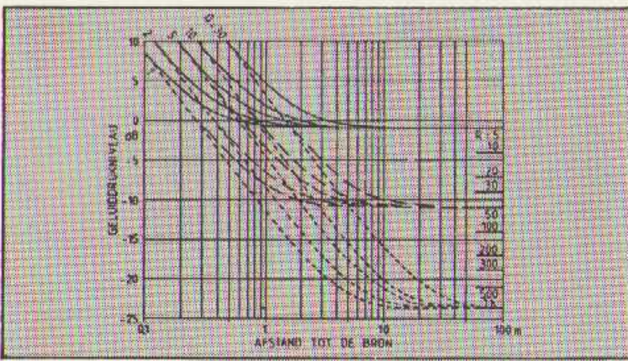
Fig. 19 Geluiddruk niveau in een kamer als functie van de afstand tot de bron, voor verschillende waarden van de richtfactor ( Q ) en de zaalkonstante ( R ). 0 dB = vermogensniveau (naar Bera- nek)
